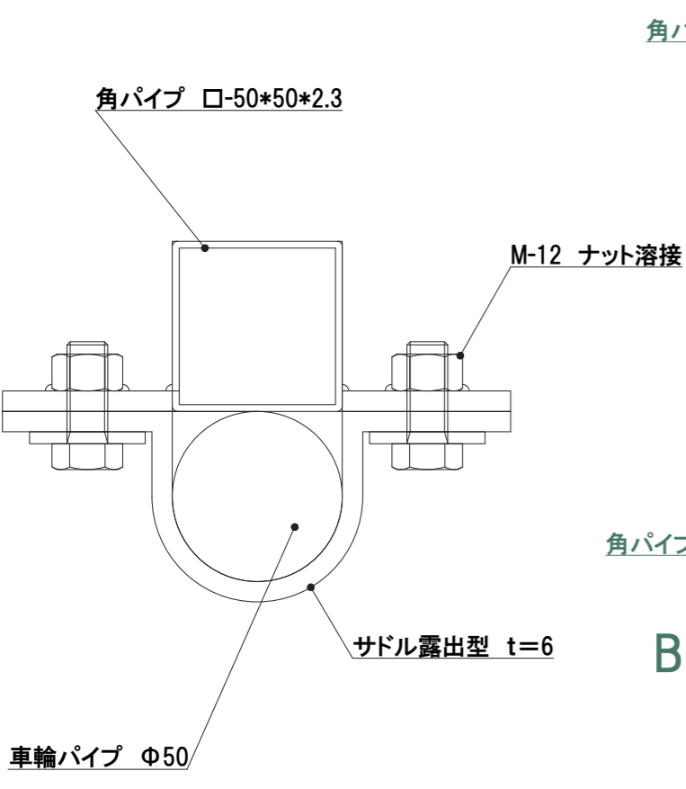
車輪部詳細図 1/2
